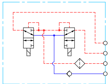
PVEO/PVEO-DI schematic
